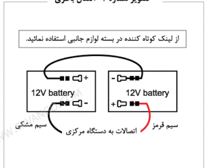
تصویر شماره ۲- اتصال باتری
